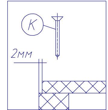
Крепление задней стенки (комплект №10)
