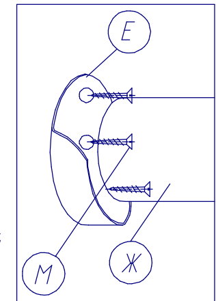
Крепление полкодержателя (комплект №8)
